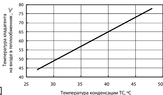
Рис. 2. Зависимость температуры хладагента на входе в теплообменник
